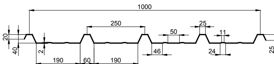
Slika 1. Kumalit krovni lim
